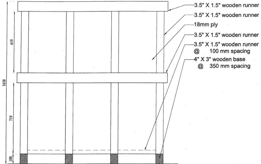
ELEVATION
